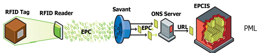
شکل ۲: اجزای سیستم RFID و نحوه ارتباط بین آنها
