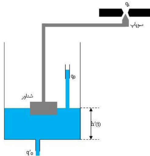
شکل ۷: سوپاپ شناور بنوموسی
