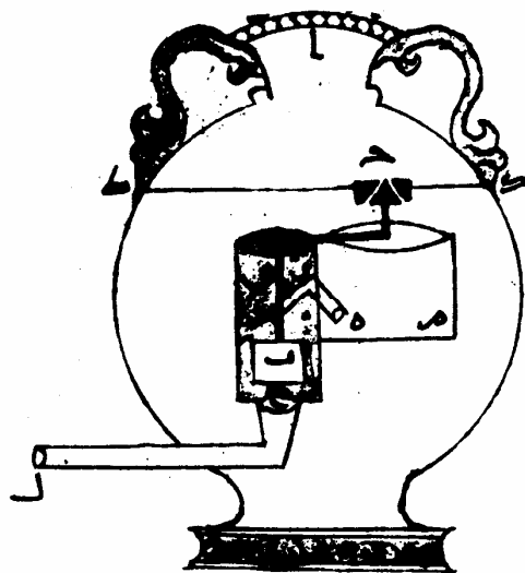
شکل ۹: نمودار طرح ۳۲ از نسخه خطی توپکاپی (۴)، ص. ۳۱۲
