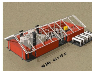
شکل ۴: اندازه سیستم VSC برای توان ارسالی ۵۰ مگاوات
