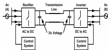
شکل ۱: سیستم HVDC
