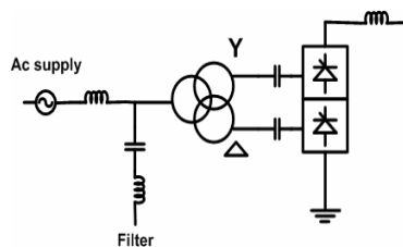
شکل ۲: سیستم HVDC با مبدل CCC
