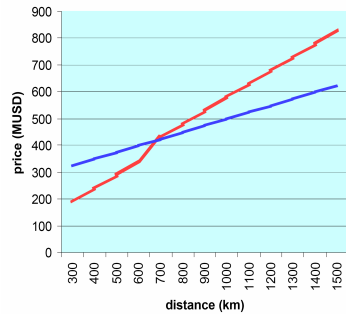
شکل ۷: مقایسه بین خط HVAC و HVDC بر حسب فاصله
