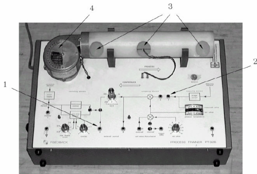
شکل ۴: سیستم Hotair dryer ( در اینجا: ۱. متغیر ورودی سیستم ۷ ، ۲. متغیر خروجی سیستم ۷ ، ۳. محل سنسورهای دما، ۴. شیر تنظیم جریان هوا)
