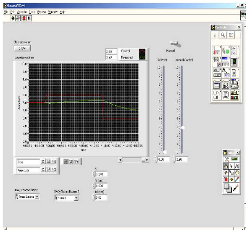
شکل ۵: صفحه نمایش طراحی شده برای پروسه حرارتی در نرم افزار LabVIEW
