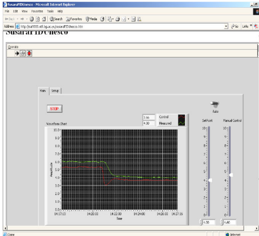
شکل ۶: صفحه نمایش برای فرایند حرارتی تحت وب
