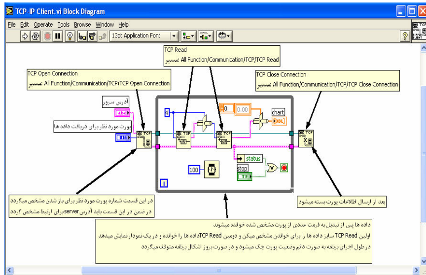
شکل پیوست ۲: برنامه Client نوشته شده برای برقراری یک ارتباط TCP/IP
