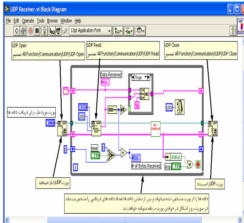
شکل پیوست ۴: برنامه گیرنده نوشته شده برای برقراری یک ارتباط UDP
