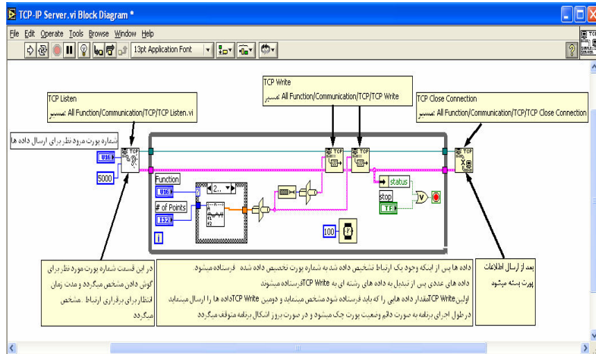
شکل پیوست ۱: برنامه Server نوشته شده برای برقراری یک ارتباط TCP/IP
