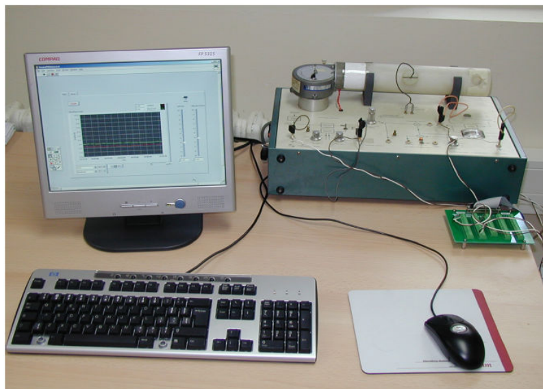
شکل ۳: سیستم فرایند حرارتی قابل کنترل از طریق وب
