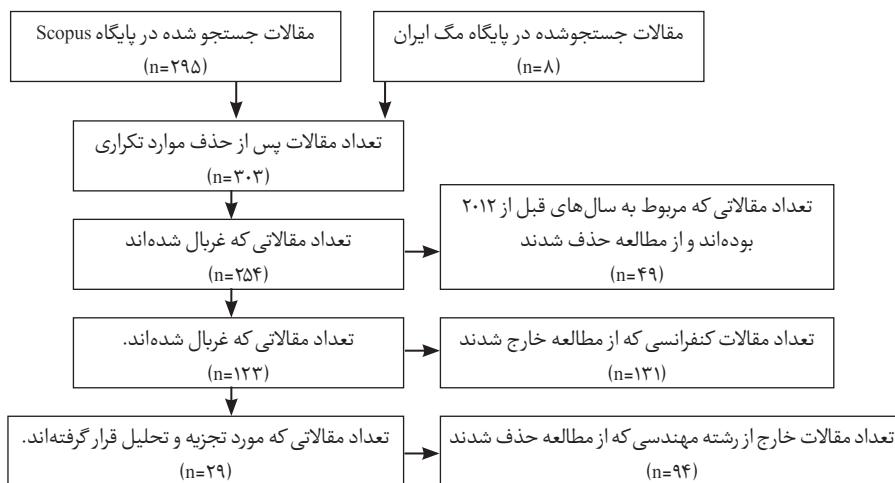
شکل ۱. نمودار پریزما
