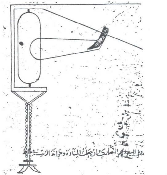
شکل ۸: تصویر شماتیک چراغ مقاوم در برابر باد
