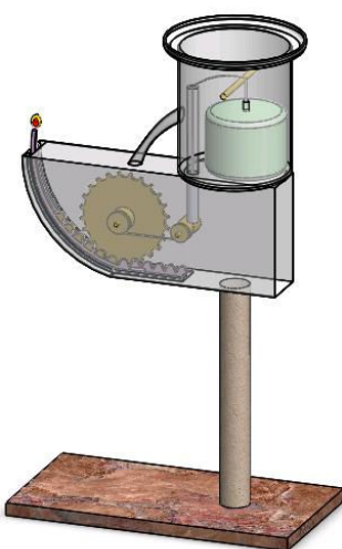
شکل ۷: تصویر کامپیوتری نمونه ساخته شده چراغ با تغذیه سوخت و تنظیم فتیله خودکار در سازمان پژوهشهای علمی و صنعتی ایران
