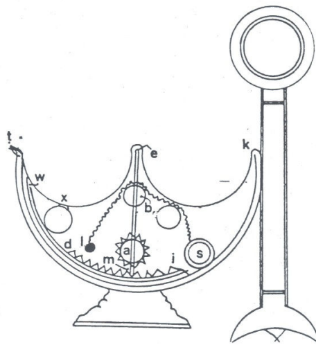
شکل ۳: تصویر شماتیک چراغ با فتیله خودتنظیم
