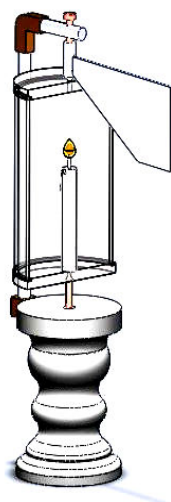
شکل ۹: تصویر کامپیوتری نمونه ساخته شده چراغ مقاوم در برابر باد در سازمان پژوهشهای علمی و صنعتی ایران
