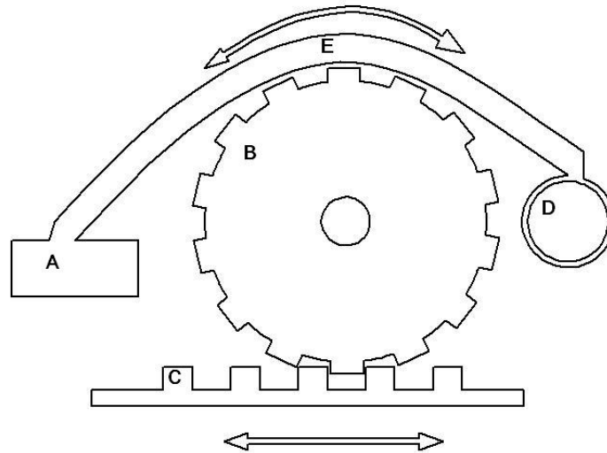
شکل ۱۱: تصویر شماتیک مکانیزم تبدیل تغییر سطح سیال به جا به جایی دورانی یا خطی با استفاده از سازکار تنظیم فتیله خودکار
